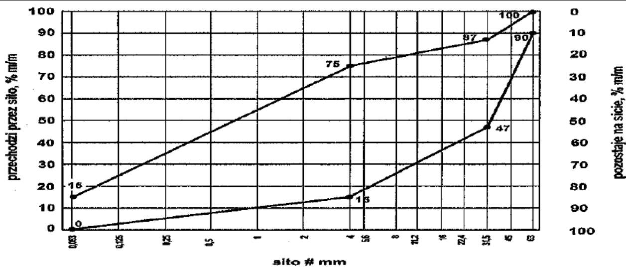
Rys. 2 Uziarnienie warstwy mrozoochronnej 0/63
