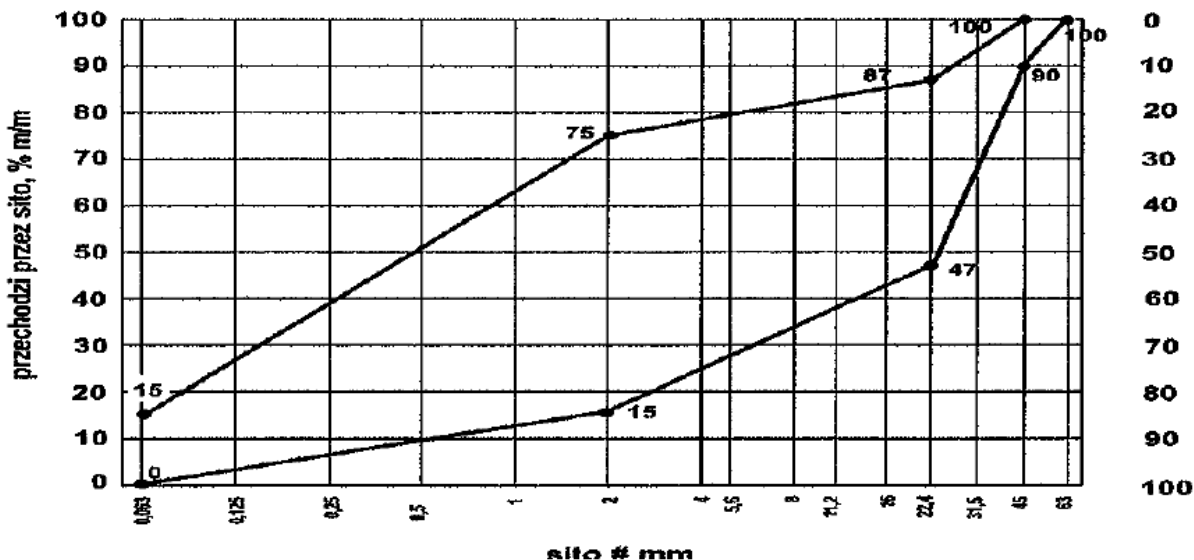
Rys. 1 Uziarnienie warstwy mrozochronnej 0/45
